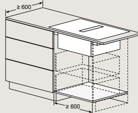
EX800NX68E, EX807NX68E, ED807HQ26E
