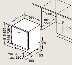
SN65T803CE Rozměry v mm
