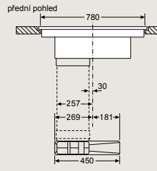
EX800NX68E, EX807NX68E, ED807HQ26E
