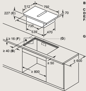
EX800NX68E, EX807NX68E, ED807HQ26E
