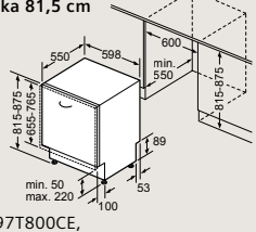
SN97T800CE, SN97T800BE, SN75Z802BE Rozměry v mm
