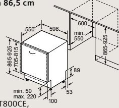
SX97T800CE, SX97T800BE, SX75Z802BE Rozměry v mm
