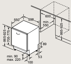
SX65T803CE Rozměry v mm
