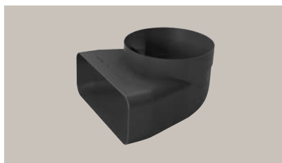
HZ9VDS11 kolenová redukce 90° pro připojení plochého potrubí a kulatých prvků potrubí o Ø 150 mm (samec)
